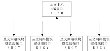
RS485 总线扩展通信模块结构示意图
