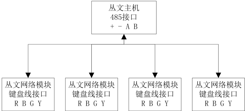
RS485 总线扩展通信模块结构示意图
